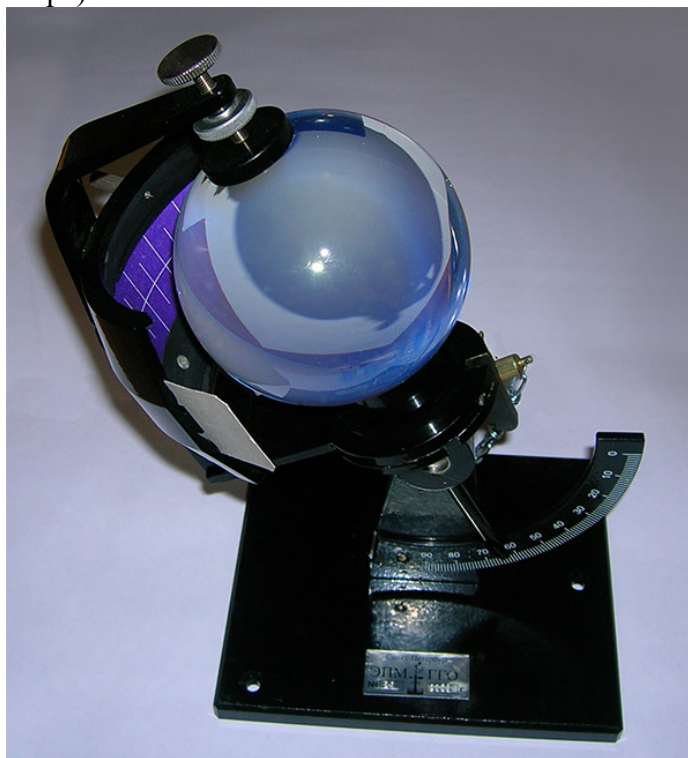
Рис. 5. Универсальный гелиограф
